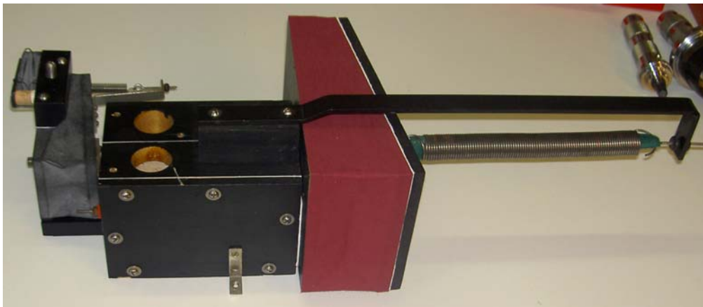
Der Klavier – Betonungsapparat nach der Restaurierung
